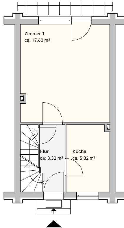
Erdgeschoss
